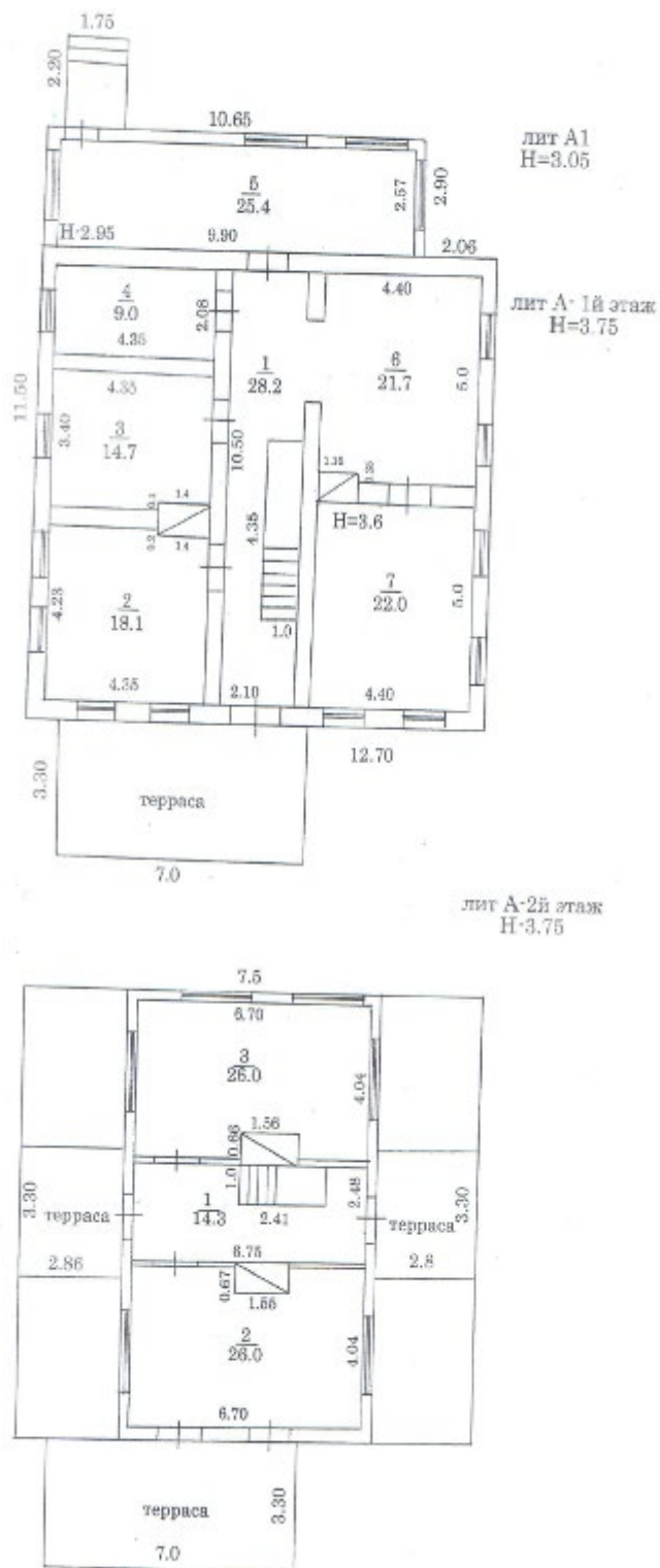
Рис.2. – Поэтажный план.
