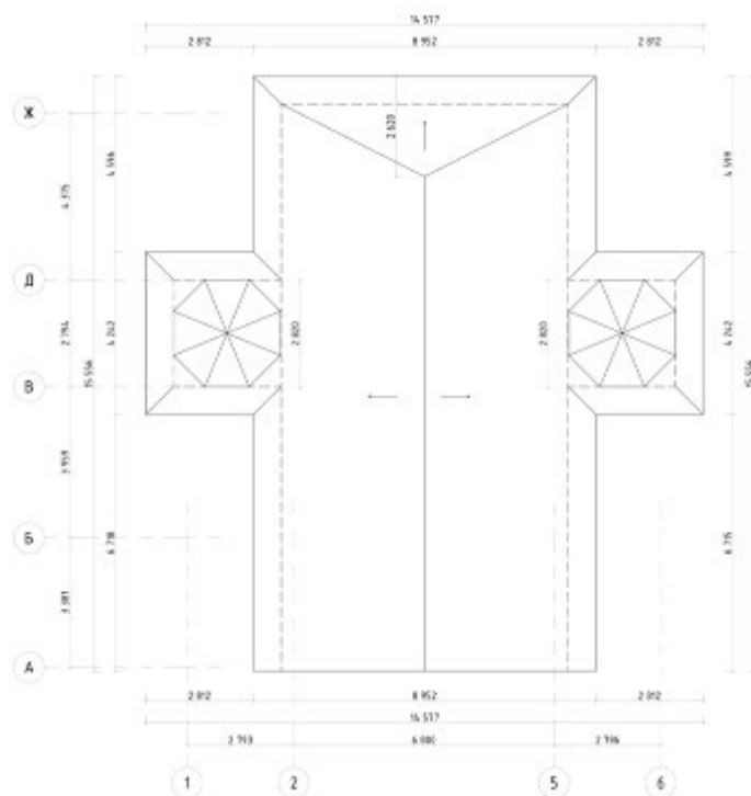
Рис.3. – План кровли.
